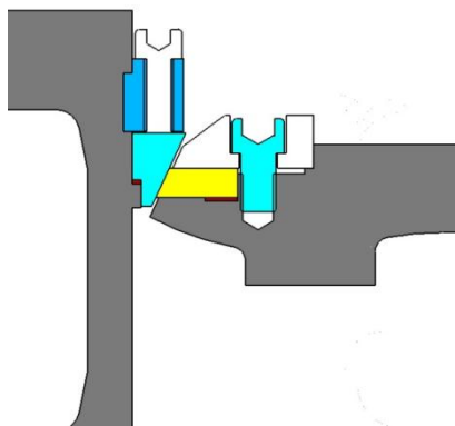
图4 双独立金属密封圈结构
