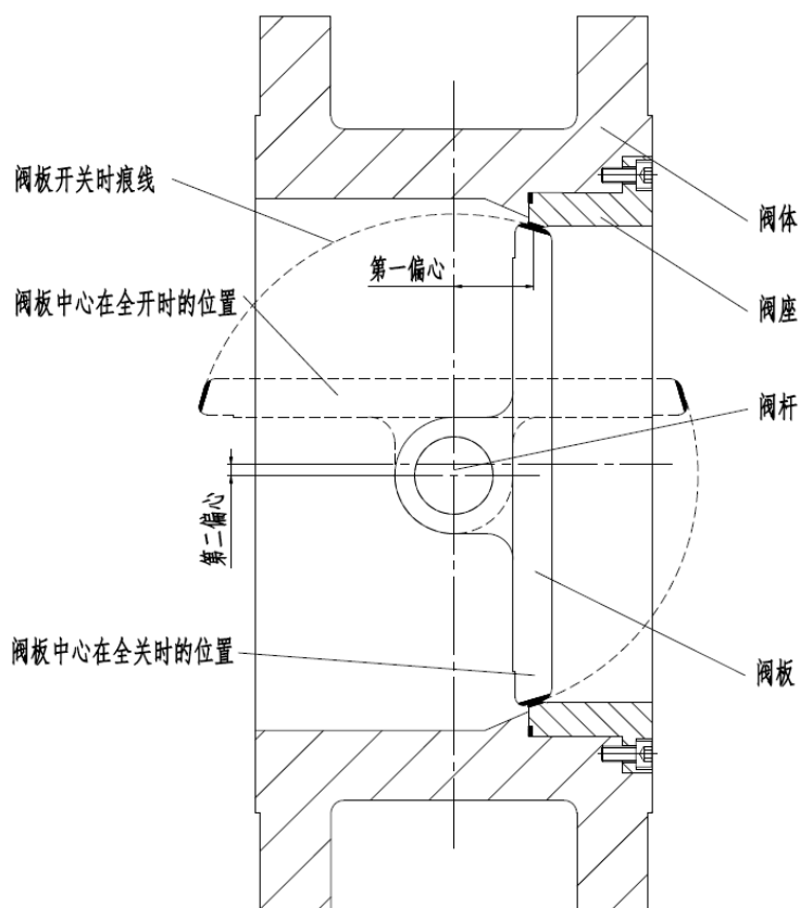
图3 双偏心原理图
