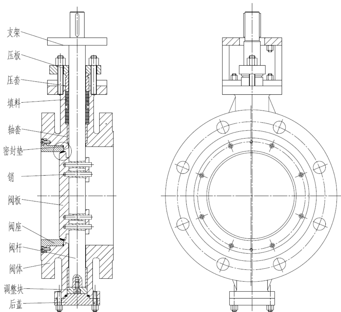
图 2 双偏心金属密封蝶阀结构图
