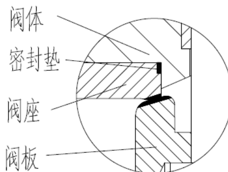
图5 单密封圈结构
