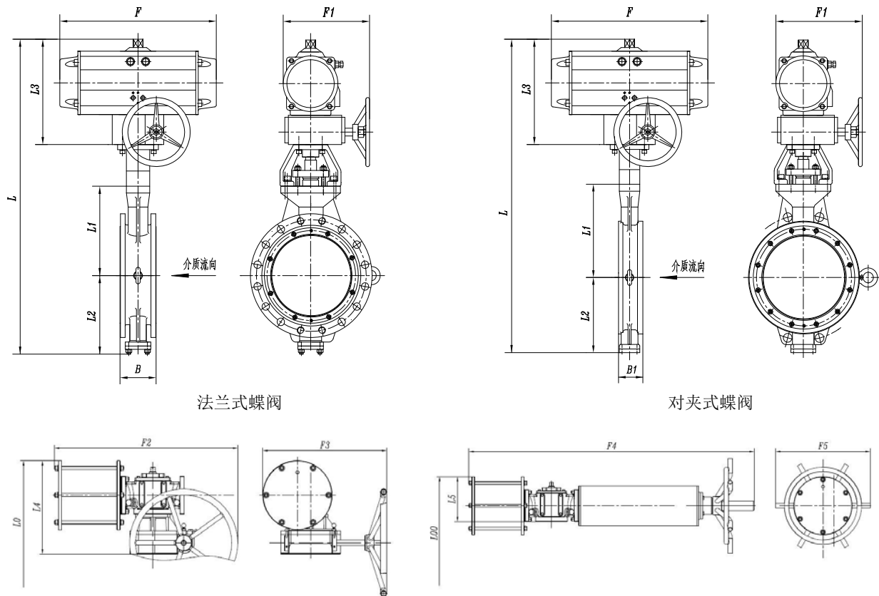
5.2 图 7： ZSH/ZSHTW 气动横推式蝶阀
