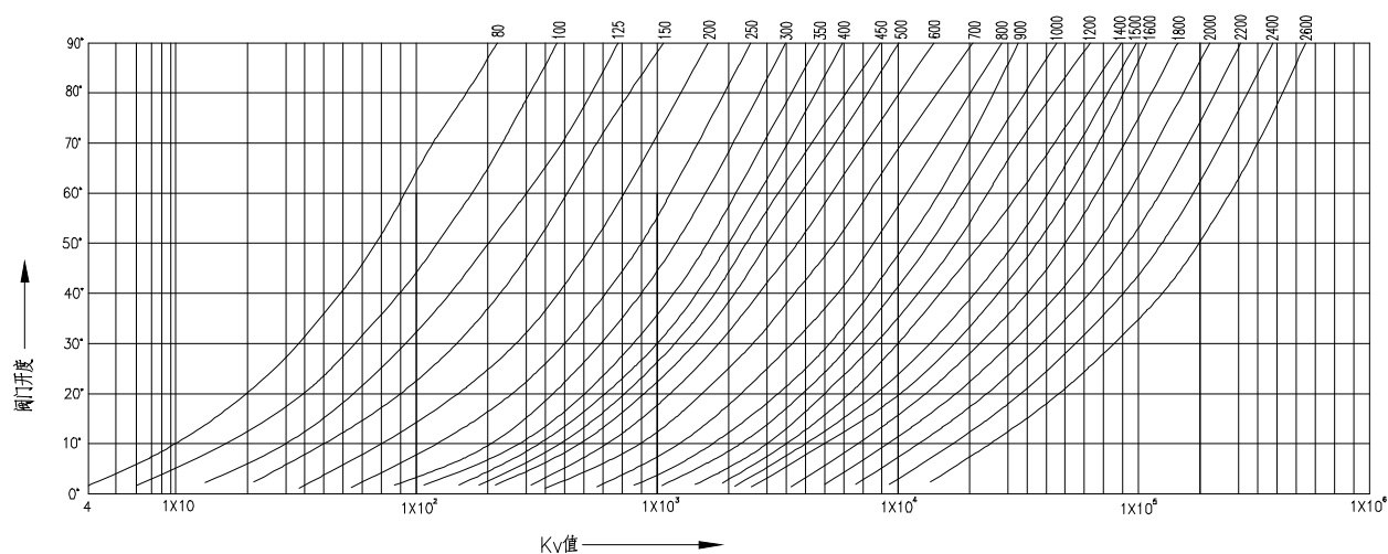
图 1 蝶阀流量特性曲线
